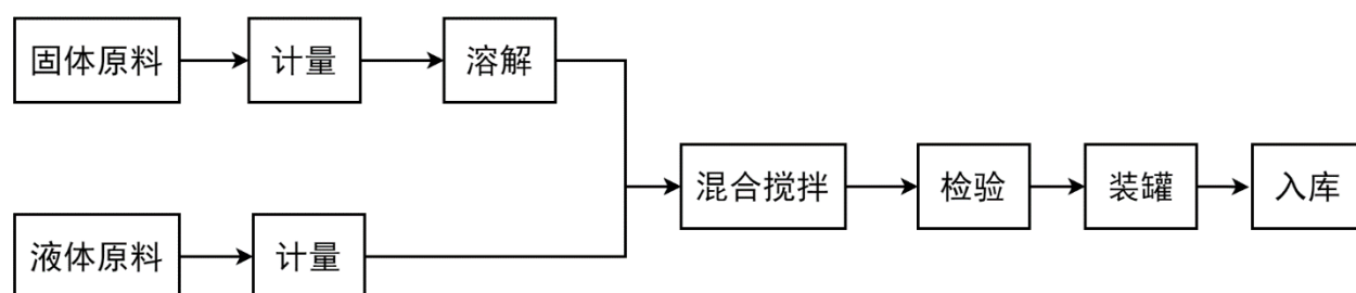
图1 玫瑰香精、檀香等（含固体原料）工艺流程图
